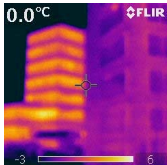
Vergleich Verwaltungsbäude Altbau (links) zu Neubau (rechts) (523, 2009)
