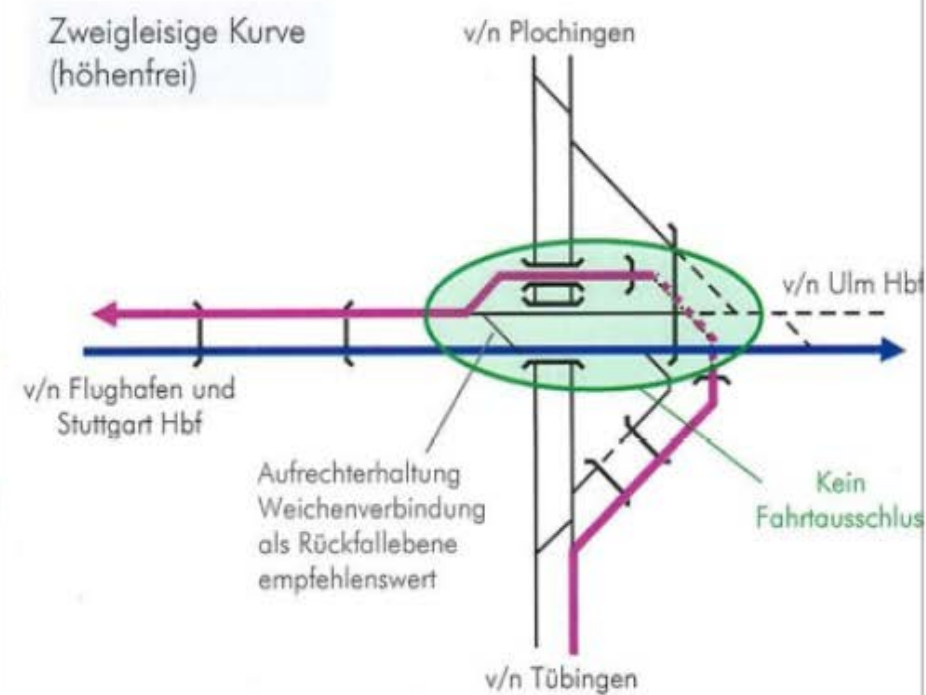
Abbildung 1: Prinzipskizze eingleisige / zweigleisige Wendlinger Kurve
