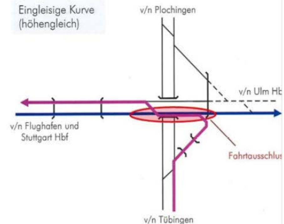
Abbildung 1: Prinzipskizze eingleisige / zweigleisige Wendlinger Kurve
